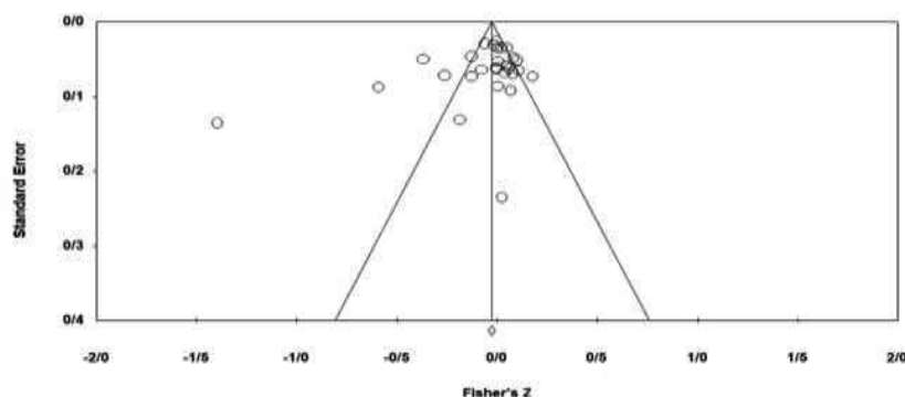
نمودار ۱. نمودار کیفی مربوط به متاآنالیز
