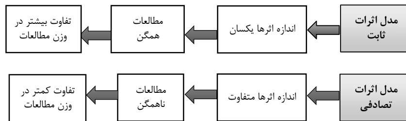
شکل ۱. ویژگی‌های مدل‌های اثرات ثابت و تصادفی
